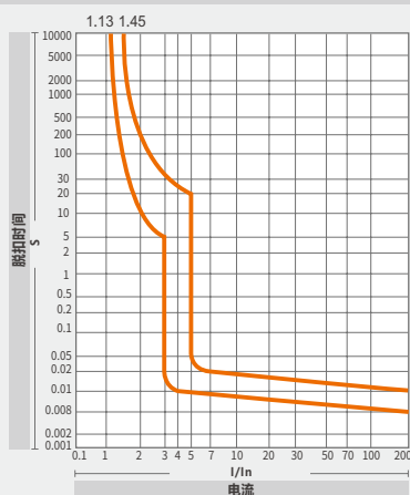
B曲线
