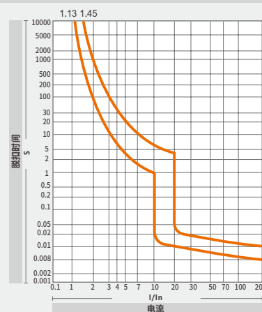
D曲线
